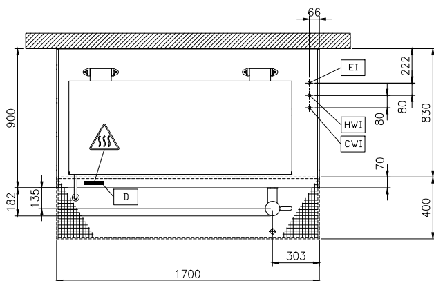
Boven aanzicht
